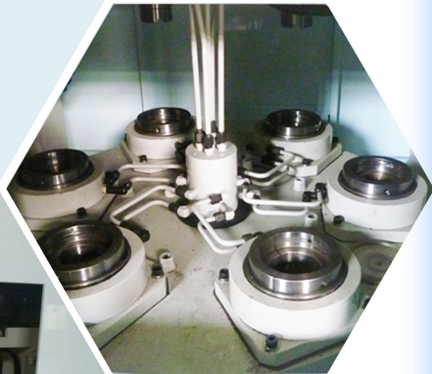
展刀軸
